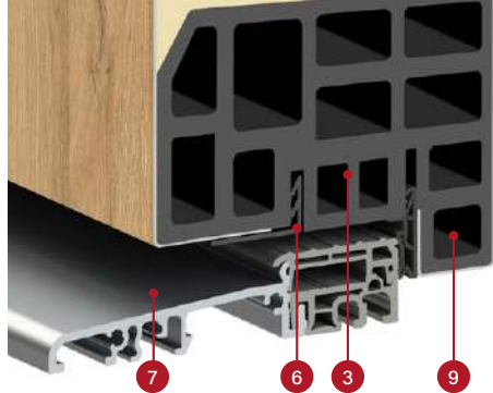
Secțiunea transversală a canatului THERMO HOT 88 cu garnitură și fără garnitură de etanșare podea, prag din aluminiu
