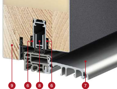
Secțiunea transversală a canatului THERMO HOT 78 cu garnitură și fără garnitură de etanșare podea, prag din aluminiu
