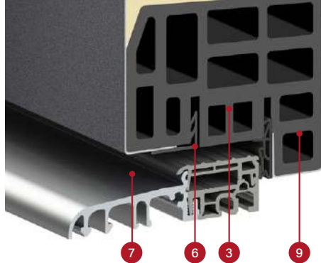
Secțiunea transversală a canatului THERMO HOT 78 cu garnitură și fără garnitură de etanșare podea, prag din aluminiu
