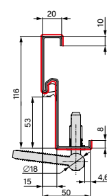
TOC DIN OȚEL DE COLȚ
