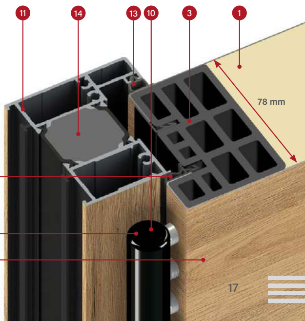
secțiunea transversală a tocului din aluminiu pentru canatul THERMO 78
